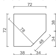
Grundriss mit den Maßen von allen Eck-Kommoden
