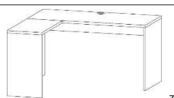
Grosse Tischplatte 135 x 61 cm Anbau-Tischplatte 74 x 40 cm
